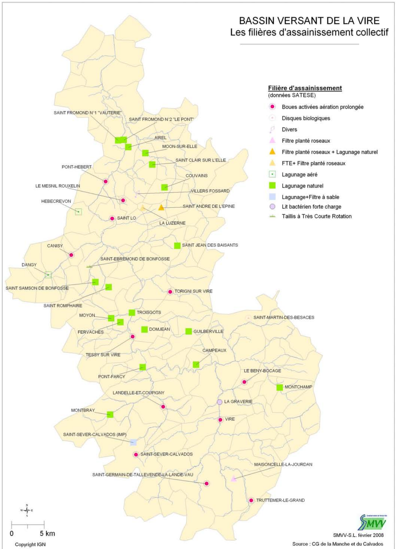
Carte 42 : Les filières d'assainissement
