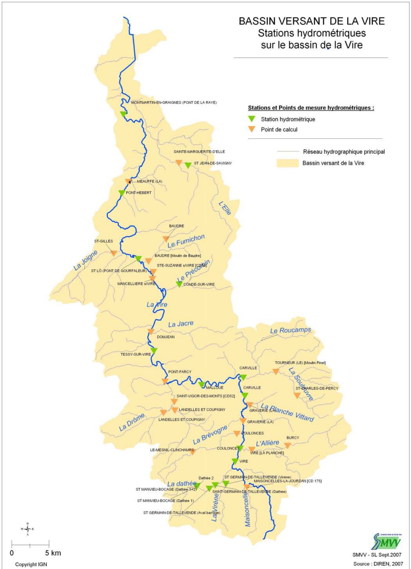
Carte 15 : Localisation des stations hydrométriques
