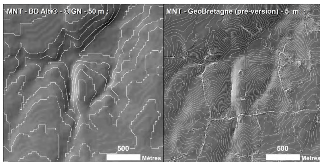
Figure 3 - Courbes de niveaux obtenues par traitements des différents MNT - à gauche équidistance 5m (MNT pas de 50 m) / à droite équidistance 1m (MNT pas de 5 m)
