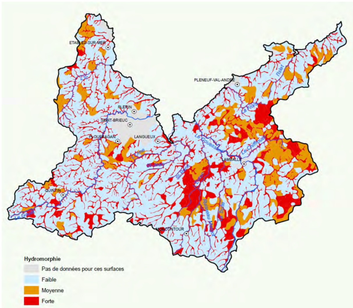
Figure 5 : Hydromorphie des sols du bassin (Etat des lieux du SAGE, 2008)
