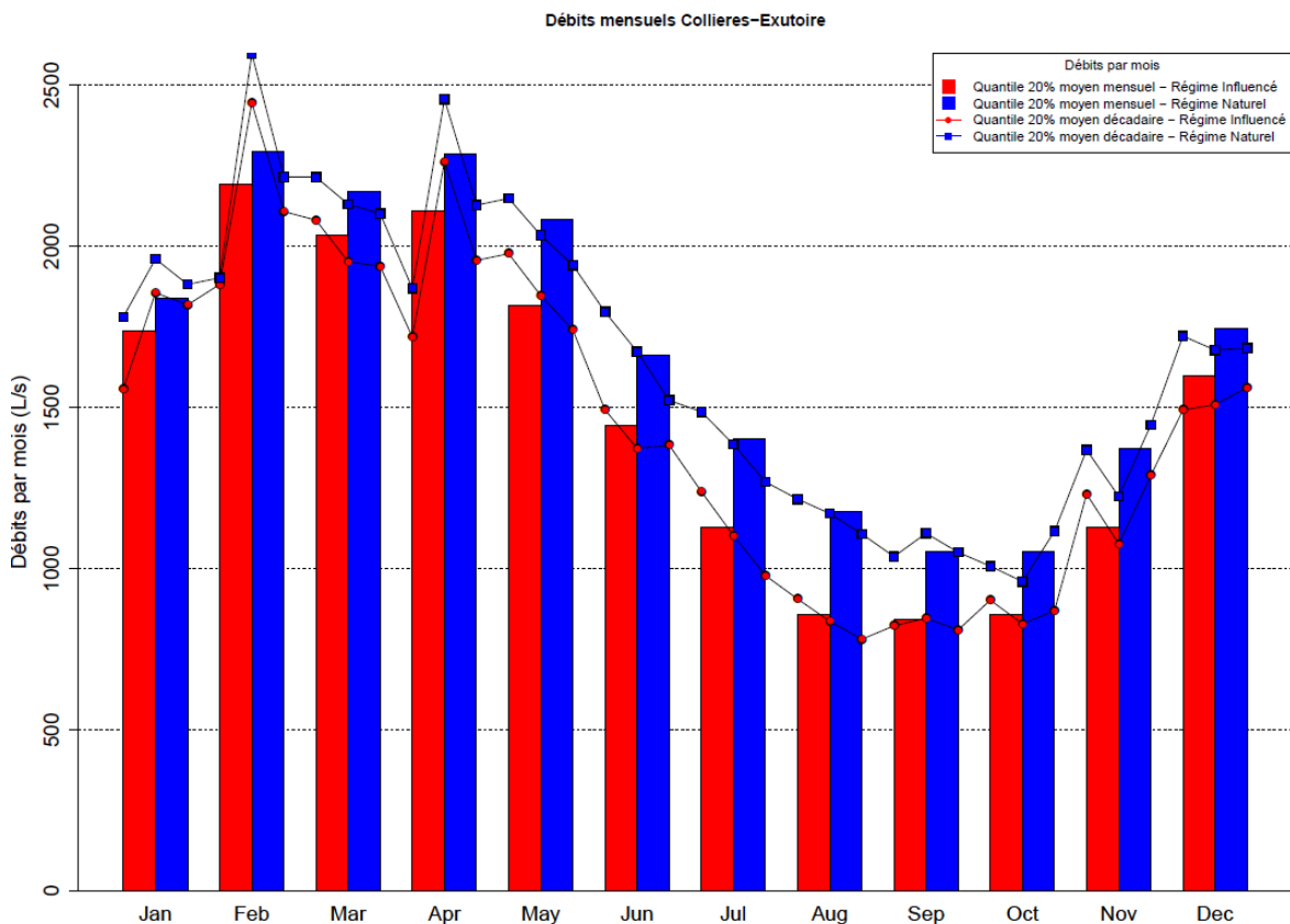
FIGURE 53 : DEBITS MOYENS MENSUELS ET DECADAIRES DES COLLIERS A ST-RAMBERT (AVAL CONFLUENCE ORON/COLLIERS) POUR UN TEMPS DE RETOUR DE 5 ANS (QUANTILE 20%)
