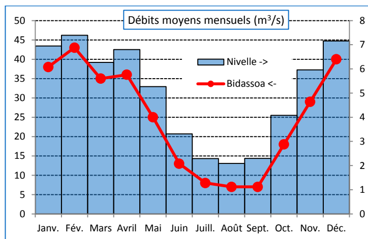
Figure 6 : Débits moyens mensuels de la Nivelle et de la Bidassoa (HydroFrance et confederation hydrographique du Cantabrique)
