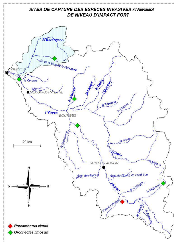
Figure 5. Carte représentant les sites de capture des espèces invasives d'impact élevé
