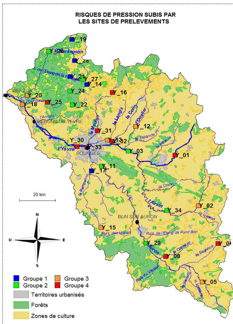
Figure 6. Carte représentant les risques de pression subis par les sites de prélèvement
