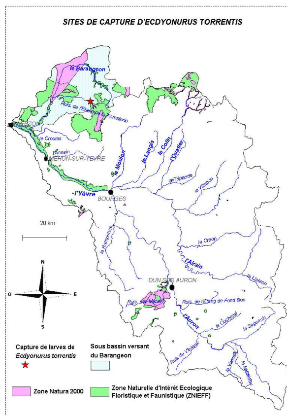
Figure 3. Carte représentant les sites de capture d' Ecdyonurus torrentis
