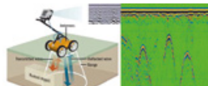
Fonctionnement du géoradar et image radar (source : CB détections)
