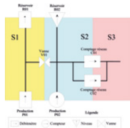
Synoptique type de la sectorisation (source : Irstea)
