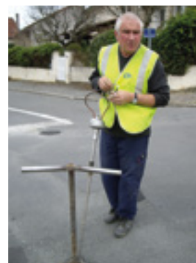
Réalisation d'une écoute directe mécanique (source : Irstea)
