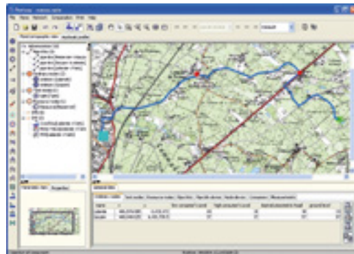
Exemple de modélisation avec le logiciel Porteau (source : Irstea)
