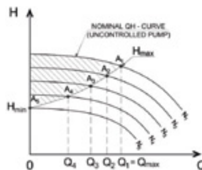
Figure B : consigne de pression variable (source : Halkijevic)
