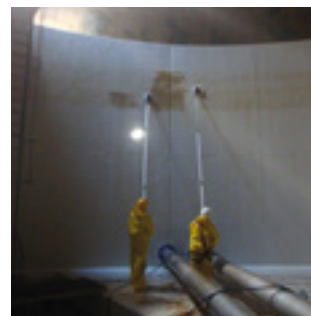
Lavage d'un réservoir (source : Herli)
