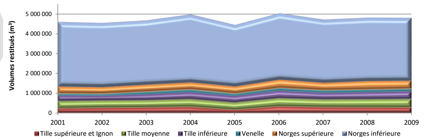
FIGURE 26: REPARTITION DES RESTITUTIONS ANNUELLES D'EAU PAR LES STEP DE 2000 A 2009 13
