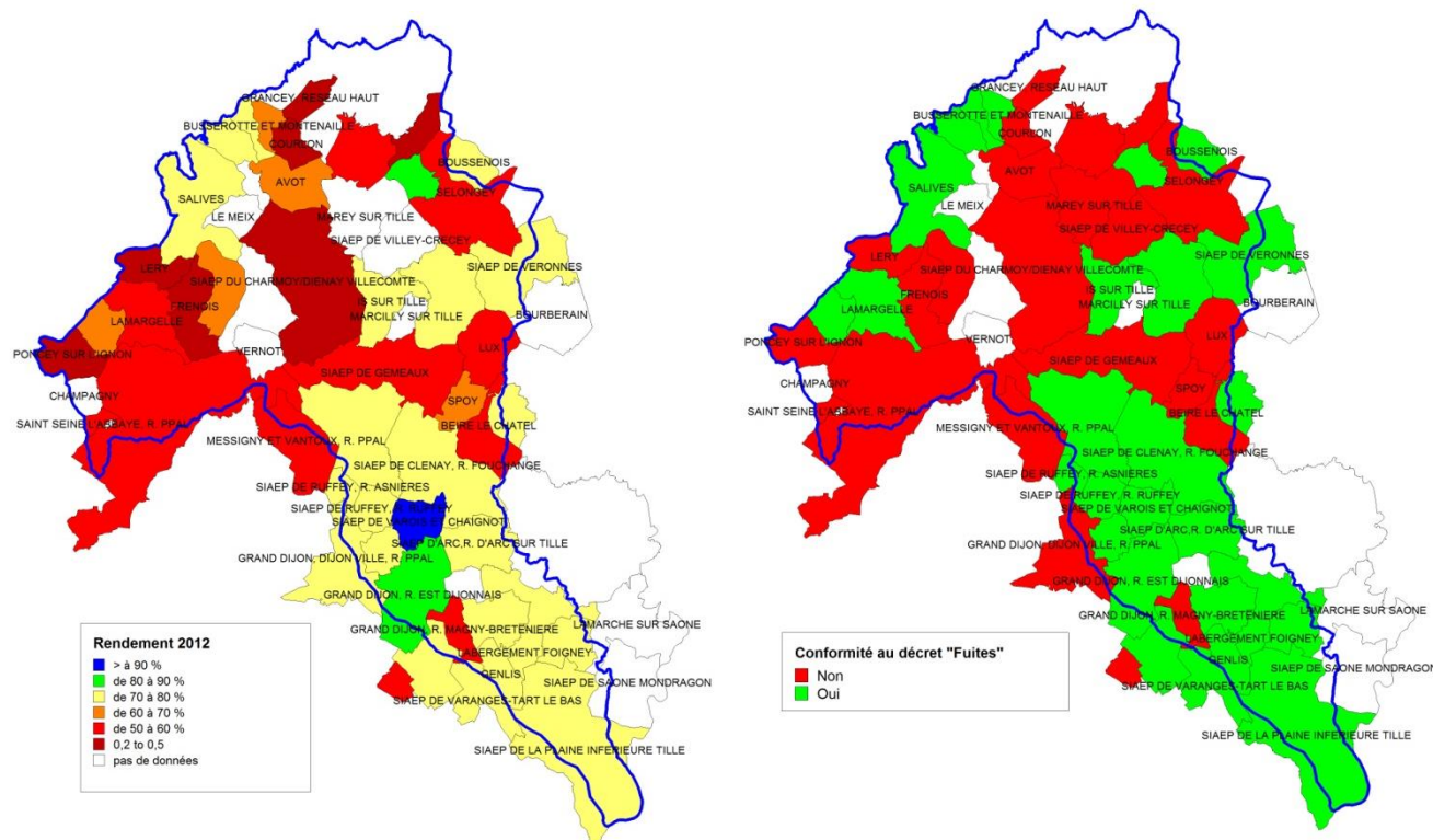
FIGURE 25: RENDEMENT CONNU DES RESEAUX AEP ET CONFORMITE AU DECRET "FUITE" EN 2012 12
