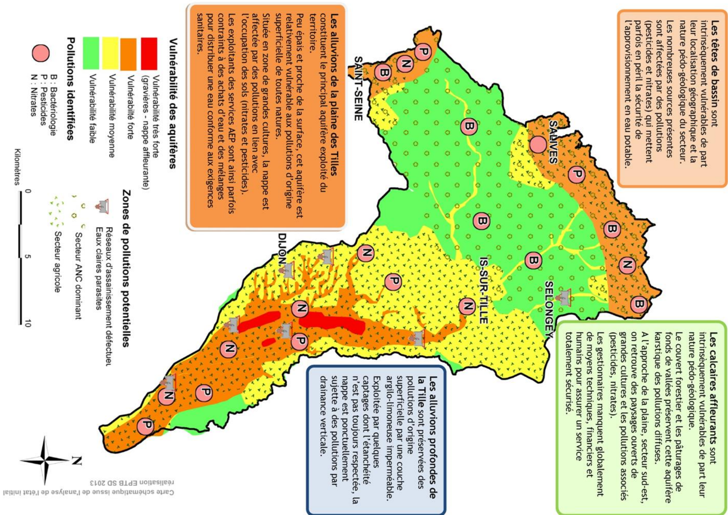
FIGURE 34: CARTE DE SYNTHESE DU DIAGNOSTIC DES PRESSIONS ET DE LA QUALITE DES EAUX SOUTERRAINES ET SUR LE BASSIN DE LA TILLE
