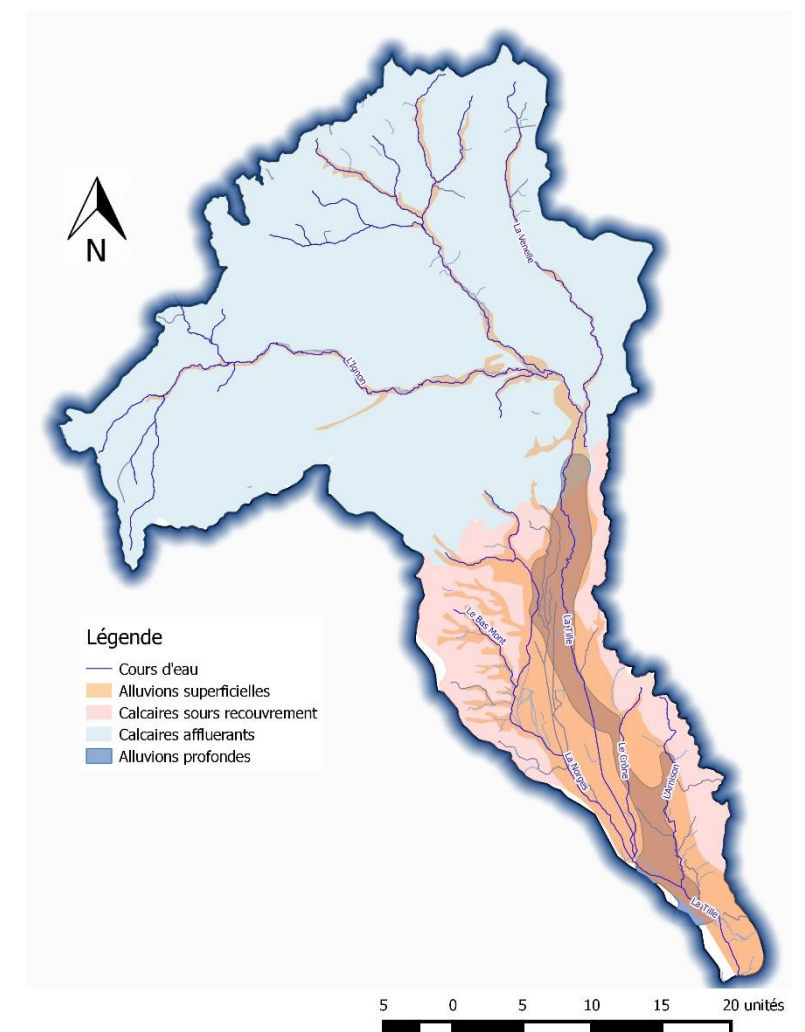
FIGURE 6: CARTE DES PRINCIPAUX COURS D'EAU ET AQUIFERES DU BASSIN
