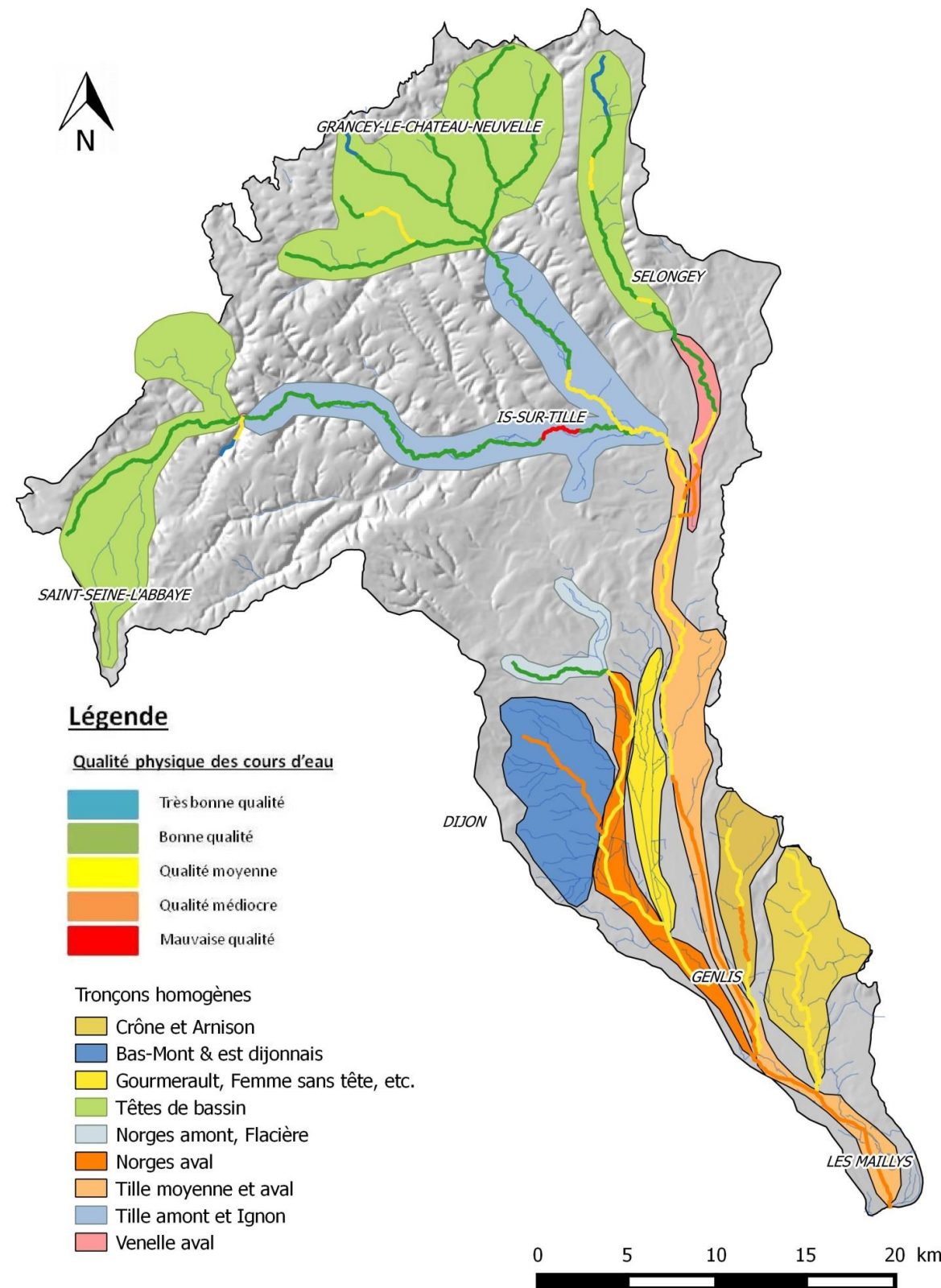
FIGURE 38: CARTE DE SYNTHÈSE DE L'HYDROMORPHOLOGIE DES PRINCIPAUX COURS D'EAU DU BASSIN DE LA TILLE
