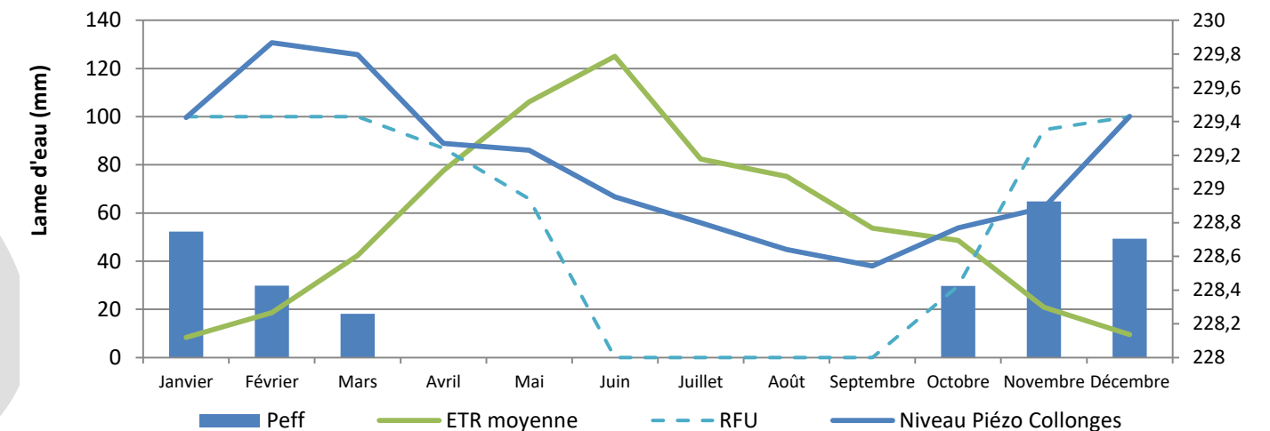
FIGURE 12: PRECIPITATIONS EFFICACES, ETP MOYENNE SUR LA PLAINE1 ET COTES NGF 2009 AU PIEZOMETRE DE COLLONGES
