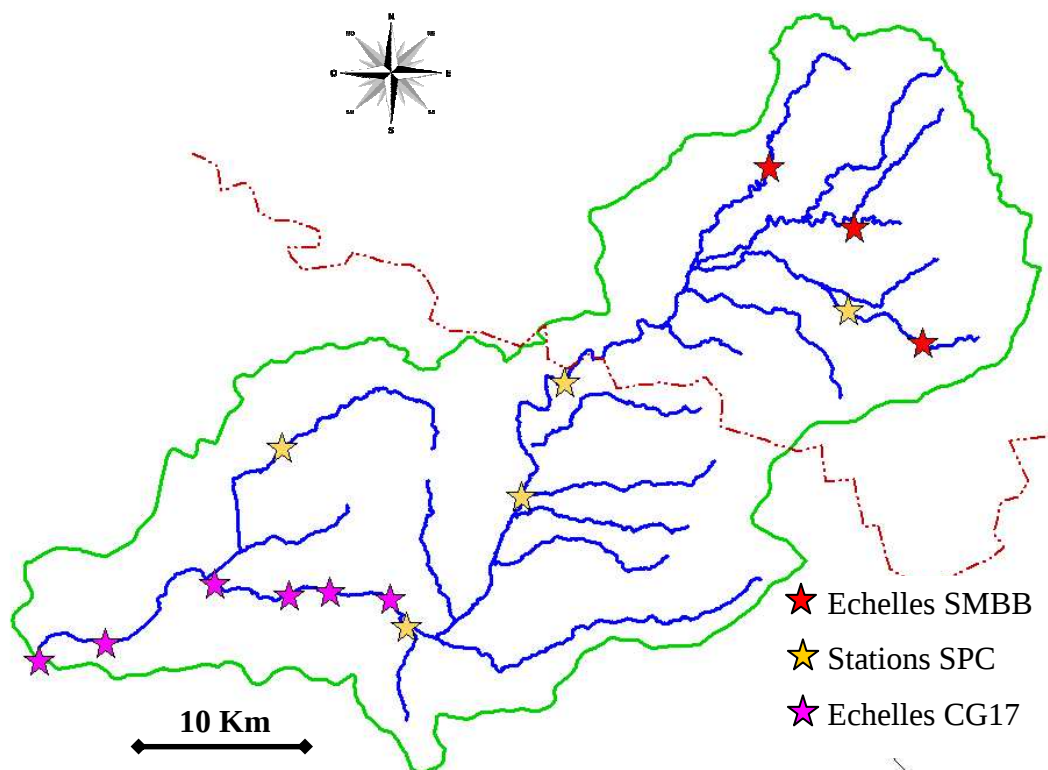
Carte 1.2 : Echelles limnimétriques suivies sur le bassin de la Boutonne en 2008
