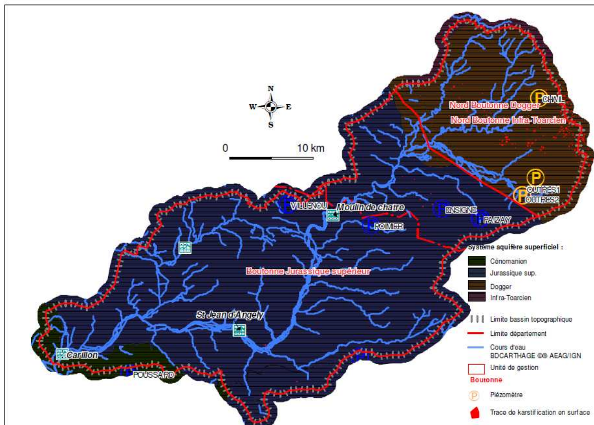
Carte 1.1 : Aquifères du bassin de la Boutonne, position des piézomètres et des stations hydrologiques, limites des zones de gestion proposées
