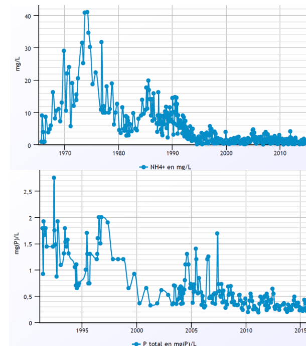
Evolution des teneurs demande biochimique en oxygène à 5 jours (DBO5), ammonium (NH4+) et phosphore total à la station de suivi Scarpe canalisée à Nivelle (01041000)
