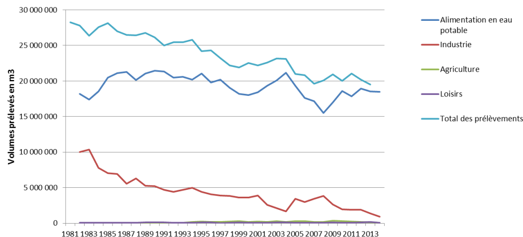
Evolution des prélèvements en eau dans la nappe de la craie de 1982 à 2014
