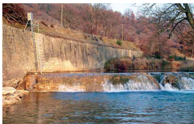
Station de mesure des débits sur le Calavon à Coste Raste
