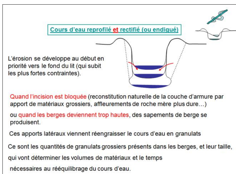
Figure 19: Processus d'érosion de berges pour les cours d'eau reprofilés et rectifiés (Source: AESN, ONEMA)
