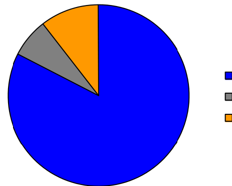
Prélèvements sur la période 2000-2014
