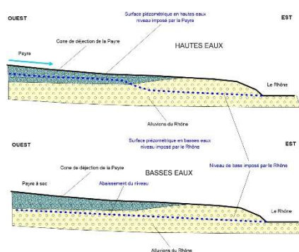
Figure 12 : coupes schématiques du fonctionnement aquifère (Idées Eaux 2011)
