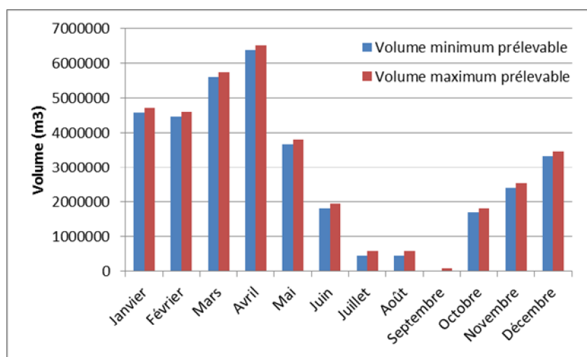
Illustration n°9 : Volume prélevable mensuel minimum et maximum (m³) à l'extrémité du bassin versant du Lez
