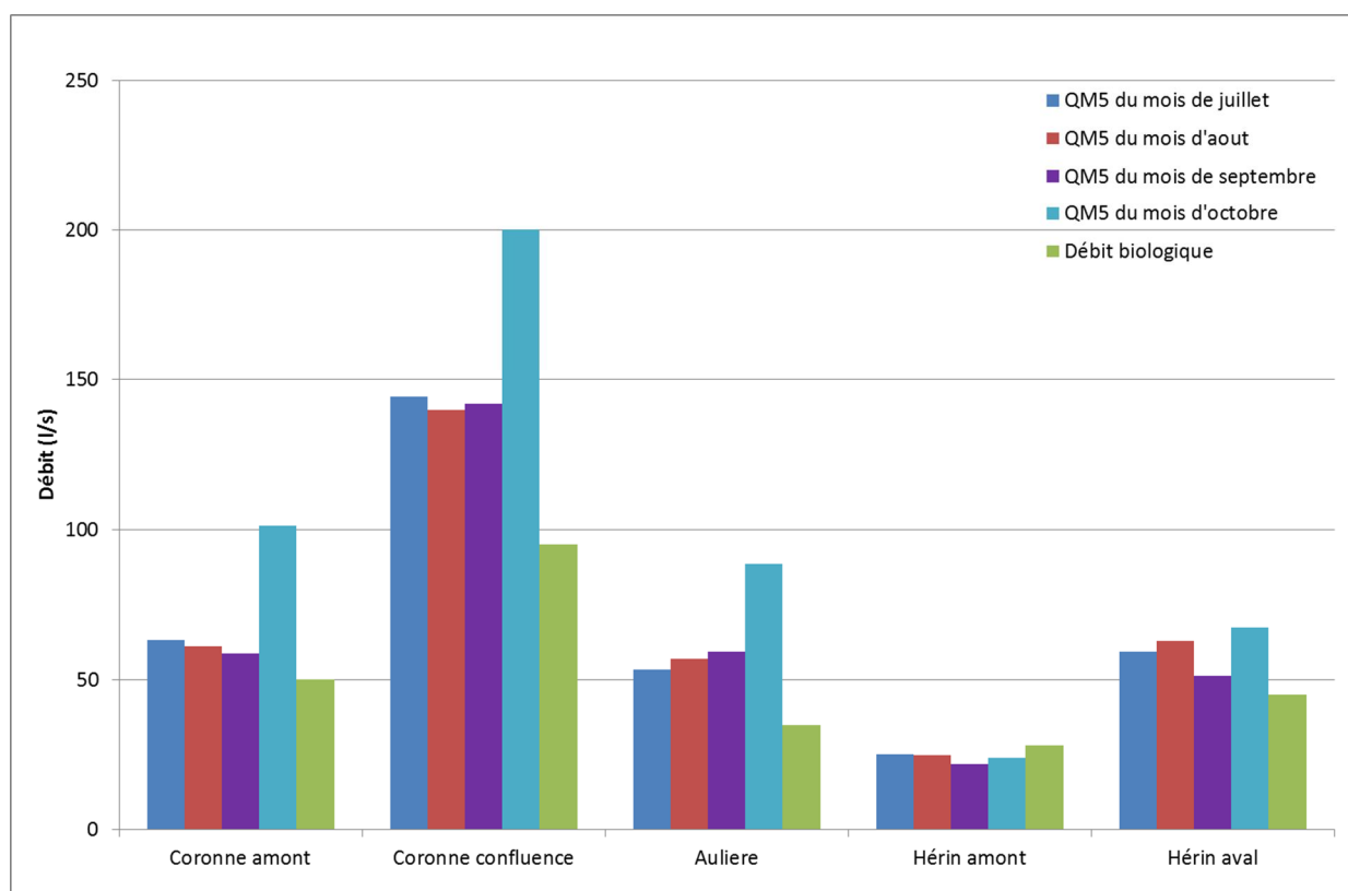
Illustration n°7 : Comparaison entre les débits caractéristiques d'entretien et les DB sur les affluents du Lez en situation naturelle
