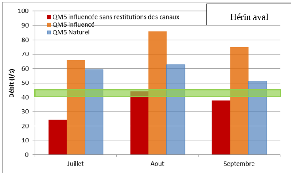
Illustration n°15 : Comparaison des QM5 sur la période d'entretien sévère sur l'Hérin aval en situation actuelle (influencée), naturelle et en situation influencée sans apports du canal du Moulin
