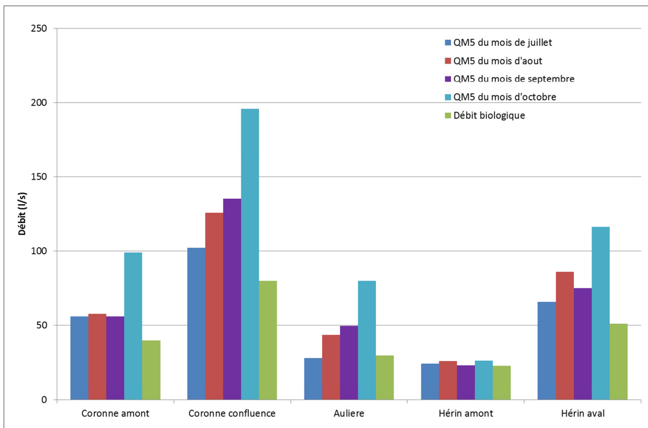
Illustration n°13 : Comparaison entre les débits caractéristiques d'œtiage et les DB sur les affluents du Lez en situation influencée
