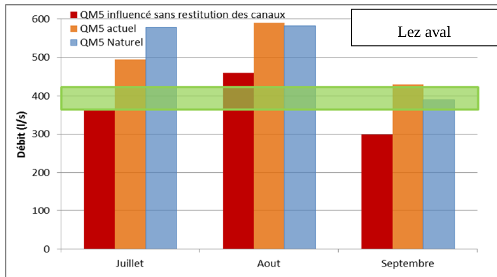
Illustration n°16 : Comparaison des QM5 sur la période d'entretien sévère sur le Lez aval en situation actuelle (influencée), naturelle et en situation influencée sans apports des canaux en amont
