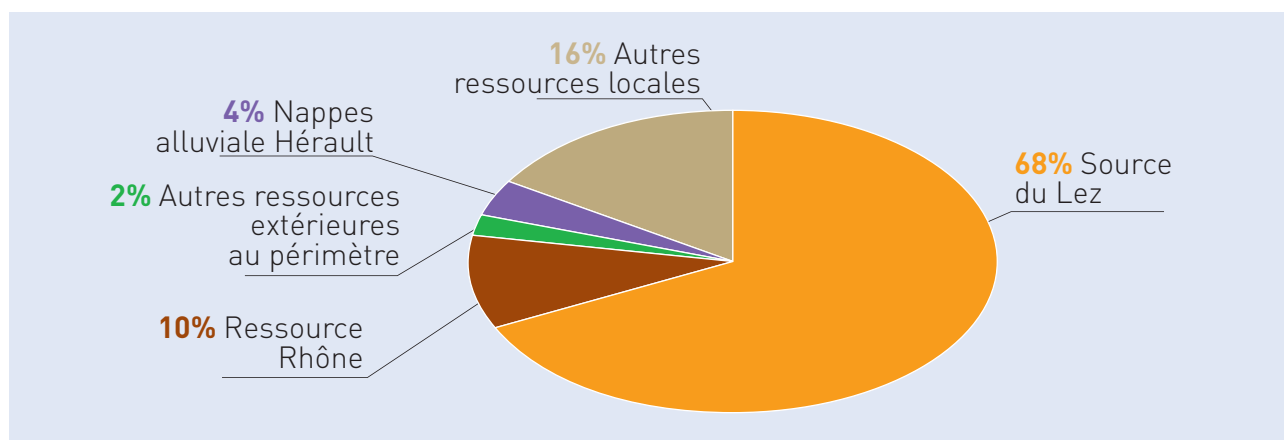
Figure n° 3 : Répartition des ressources utilisées pour l'AEP sur le périmètre du SAGE
