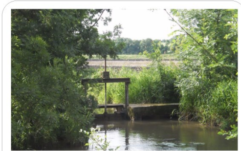
Ouvrage n° 31: Vanne Caractéristiques de l'ouvrage : Longueur : 1 m Largeur : 5 m Hauteur : 1,8 m Gestion : publique
