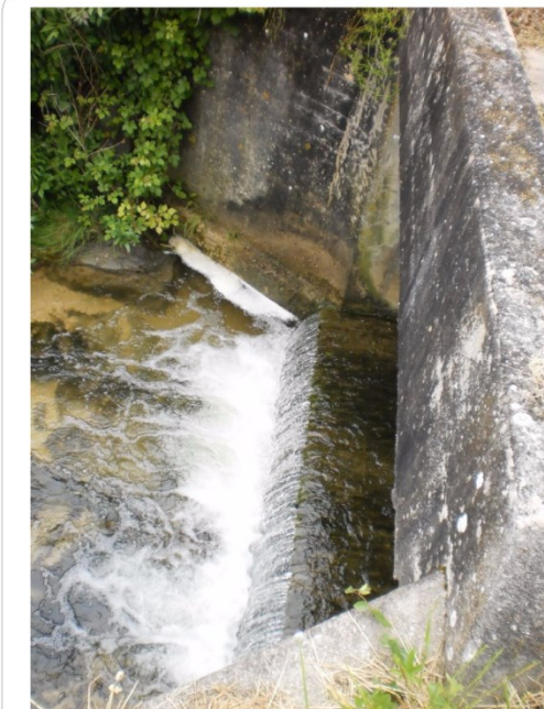
Ouvrage n° 10 : Ouvrage à madrier Caractéristiques de l'ouvrage : Longueur : 0,50 m Largeur : 3 m Hauteur : 1,2 m Etat : Abandon
