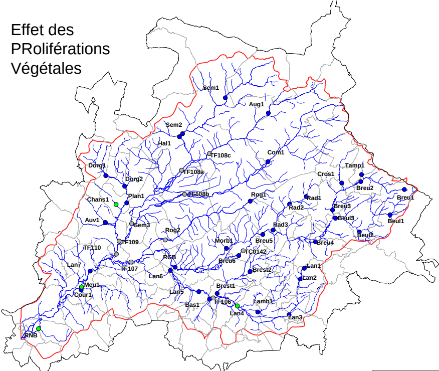
Indice Biotique Global Normalisé
