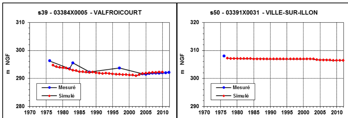
Figure 6 : Niveaux mesurés et simulés de 1977 à 2010 – Secteur sud-est du SAGE (Valfroicourt-Ville-sur-Illon).
