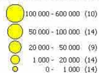
Prélèvements AEP en été en 2002 (en m3)
