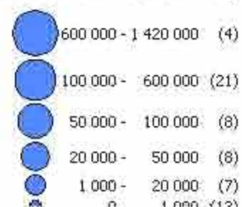
Prélèvements AEP annuels en 2002 (en m3)
