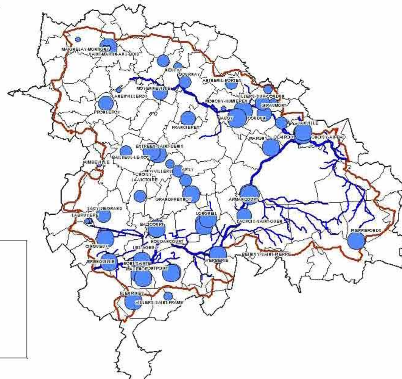
Prélèvements AEP annuels en 2002 (en m3)
