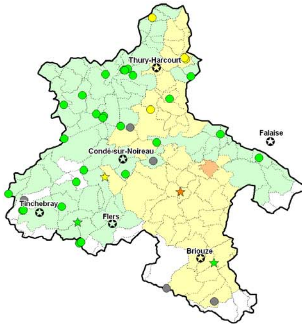
Teneurs maximales en atrazine et déséthylatrazine dans les eaux distribuées en 2000-2001
