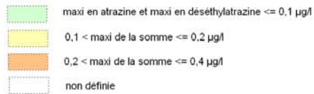
Concentrations maximales en atrazine ou déséthylatrazine en 2000-2001 dans les eaux souterraines
