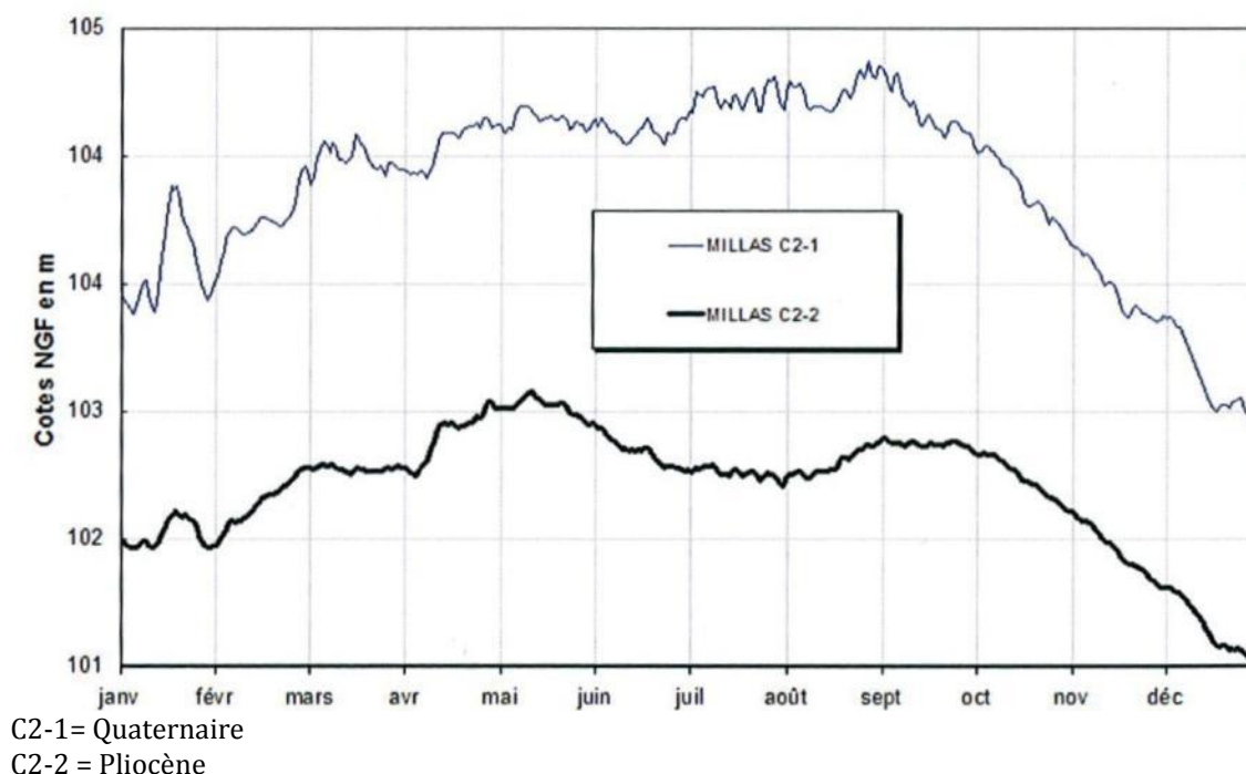
Figure 42 : Suivi piézométrique 2009 des nappes Quaternaire et Pliocène à Millas (source BRGM-SMNPR)
