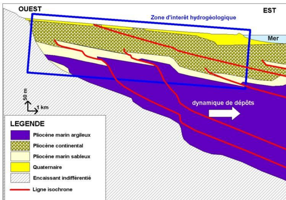
Figure 23 : Coupe géologique schématique de la plaine du Roussillon (reprise simplifiée de la coupe dressée par B. Aunay dans le cadre de ses travaux de recherche - 2007)
