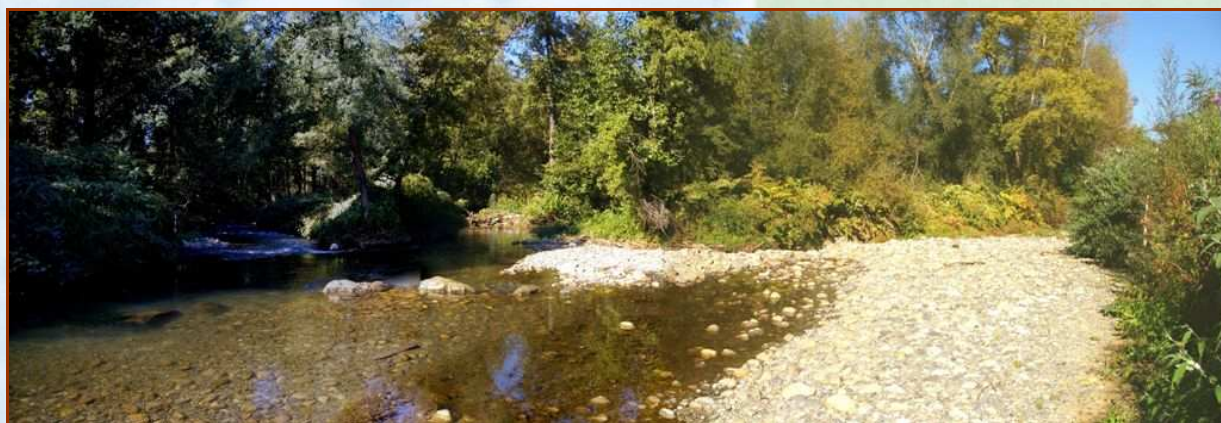
Octobre 2011 : changement de lit de l'Adour à Horgues
