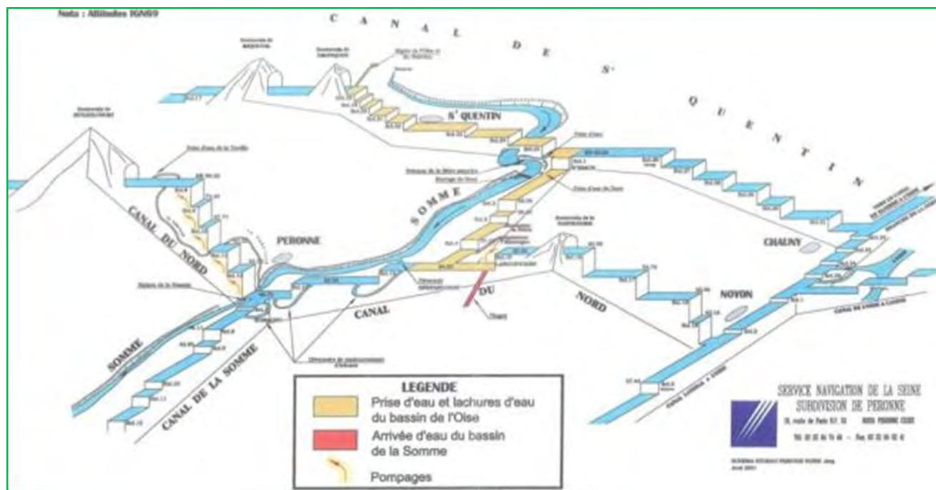
Schéma 10 : Fonctionnement hydraulique de la Somme amont (VNF)
