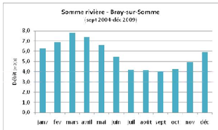
Graphique 5 : Débits mensuels moyens de la Somme rivière à Bray-sur-Somme
