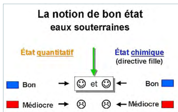
Schéma 3 : La notion de bon état des eaux
