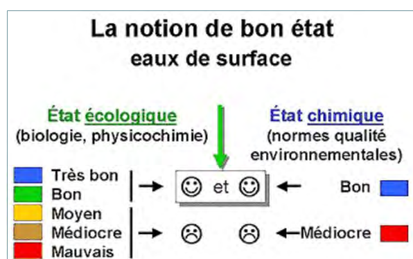
Schéma 9 : Bon état des eaux superficielles (FNE)
