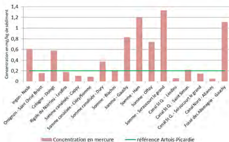
Graphique 4 : Concentration en mercure dans les sédiments en 2013 (AEAP)
