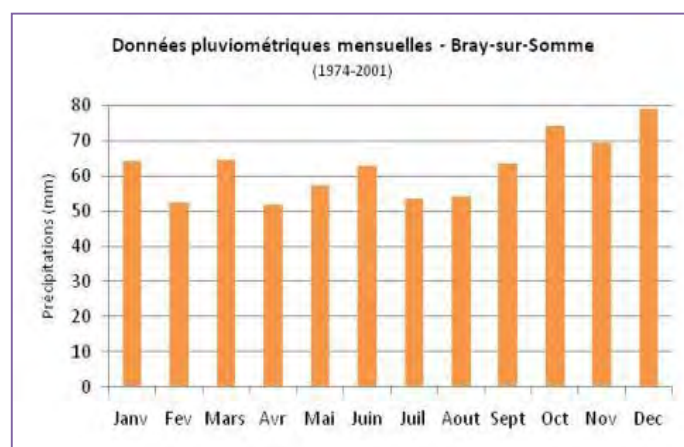
Graphique 1 : Pluviométrie moyenne mensuelle - Bray sur Somme - 1974/2002 (MétéoFrance)
