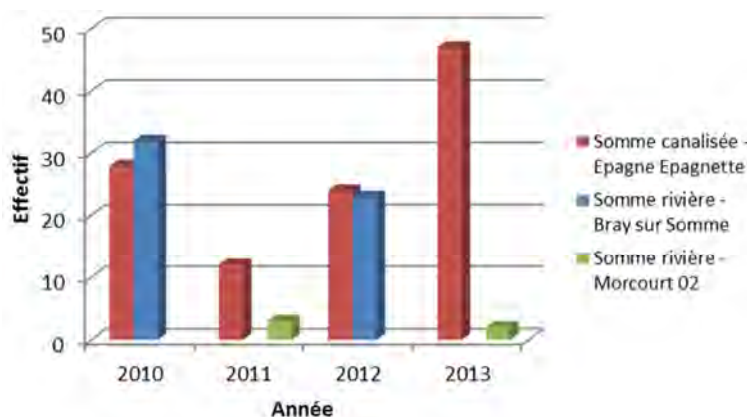
Graphique 8 : Effectifs d'anguilles entre 2010 et 2013, de l'aval à l'amont sur la Somme (ONEMA)
