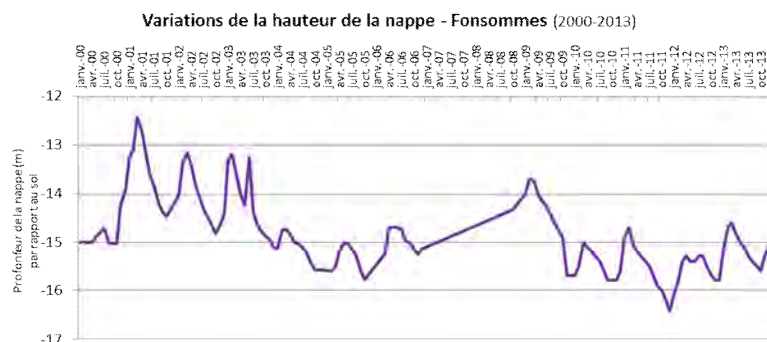
Graphique 2 : Variations moyennes mensuelles de la hauteur de la nappe au niveau de Fonsomme de 2000 à 2013 (AEAP)
