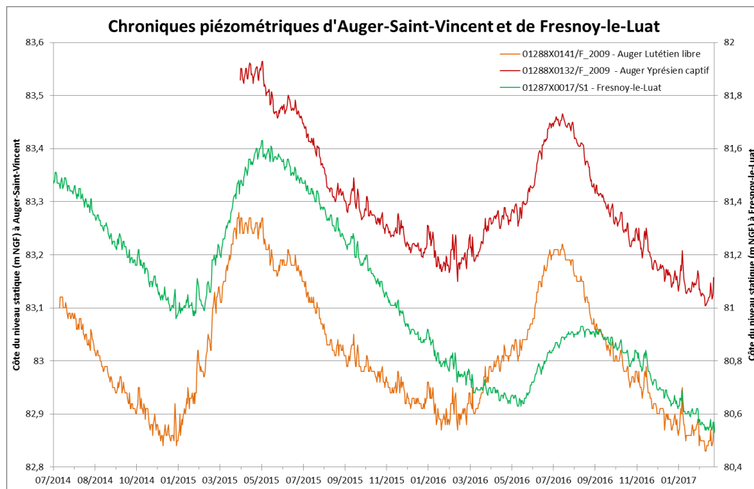
Figure 3 : Chroniques piézométriques des ouvrages d'Auger-Saint-Vincent et de Fresnoy-le-Luat
