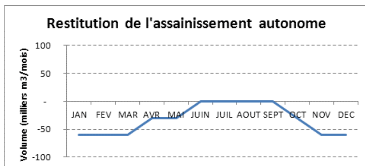
Figure 24 : restitution mensuelle de l'assainissement autonome sur le bassin de l'Ouche
