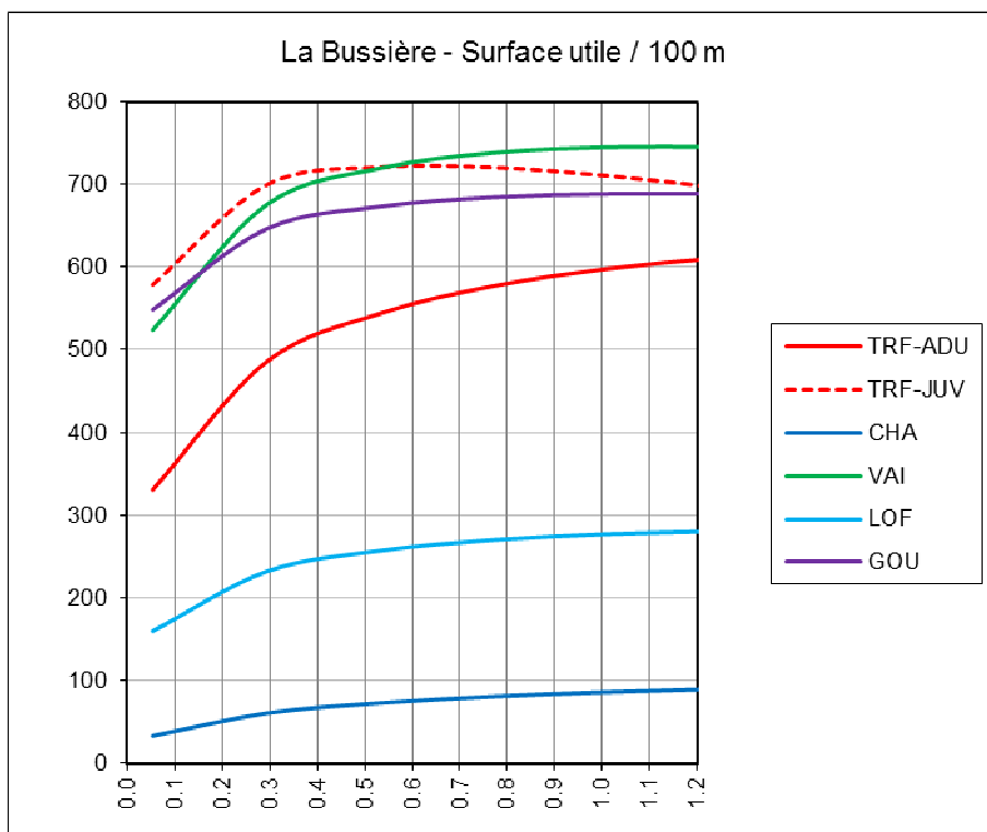
Figure 19 : La Bussière – Valeur d'habitat et surface utile par espèce (surface utile en m²/100 m en fonction du débit en m³/s)
