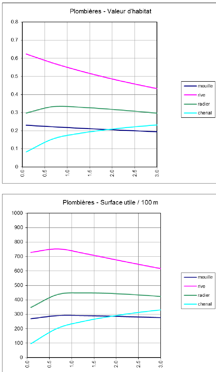
Figure 25 : Plombières – Valeur d'habitat et surface utile par guildes (surface utile en m^2/100\ m en fonction du débit en m^3/s )
