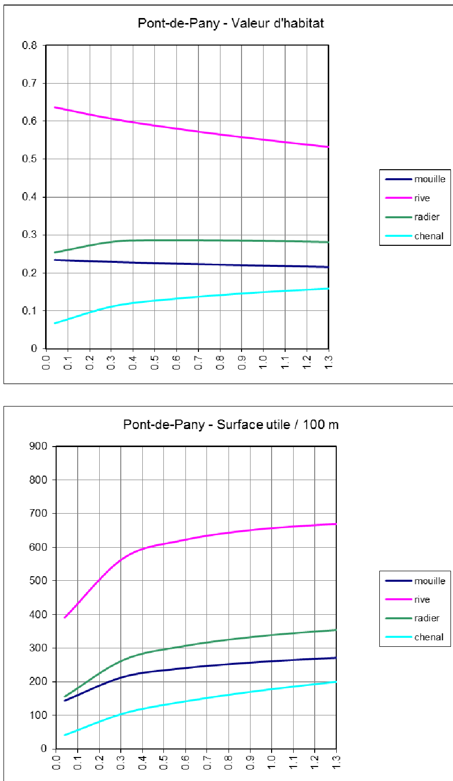
Figure 23 : Pont-de-Pany – Valeur d’habitat et surface utile par guildes (surface utile en m²/100 m en fonction du débit en m³/s)
