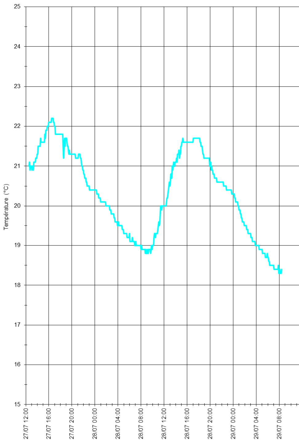
Figure 3 : Crimolois – Variations nycthémérales de la température – Juillet 2003
