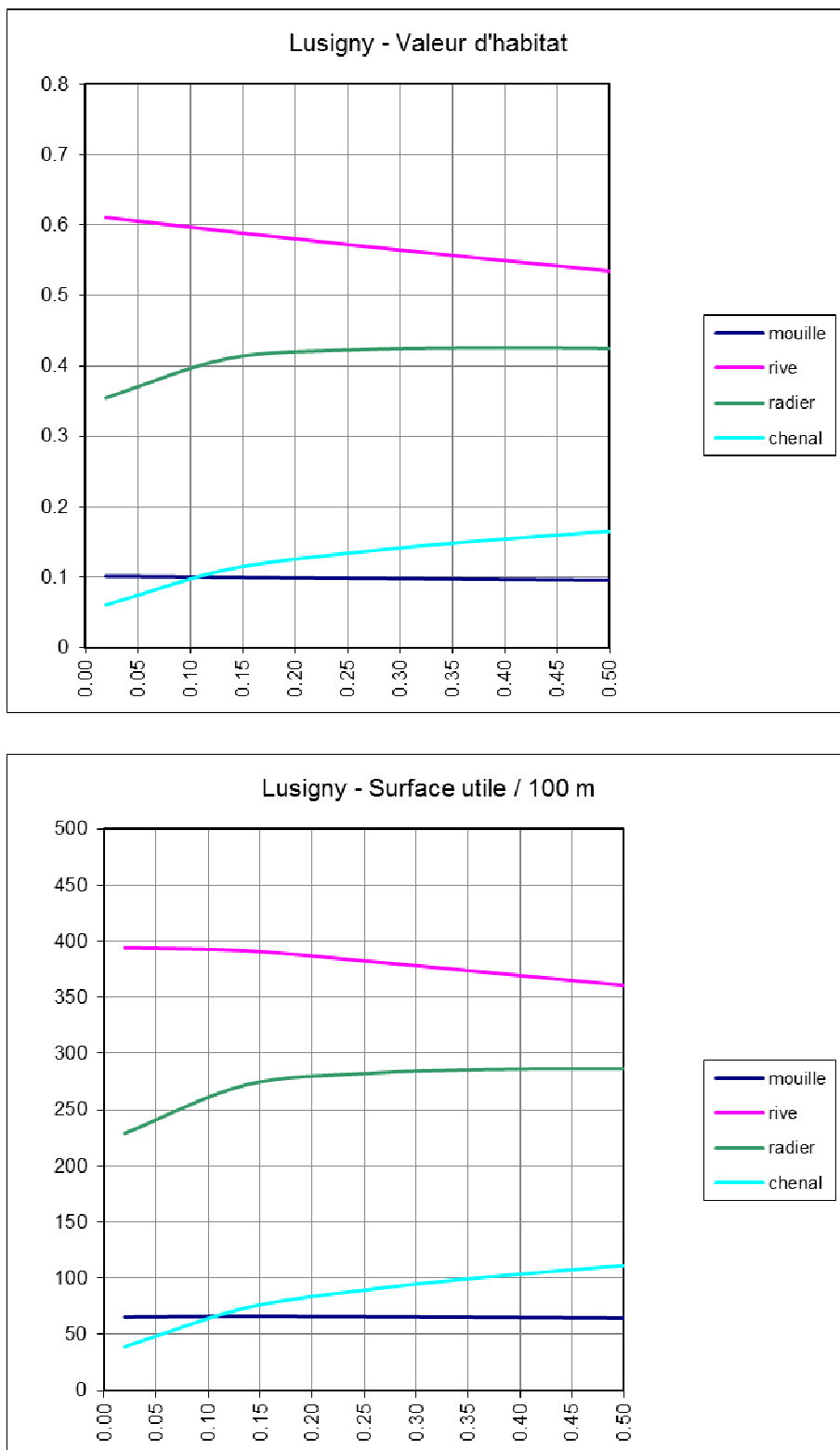
Figure 15 : Lusigny – Valeur d’habitat et surface utile par guild (surface utile en m^2/100 m en fonction du débit en m^3/s )
