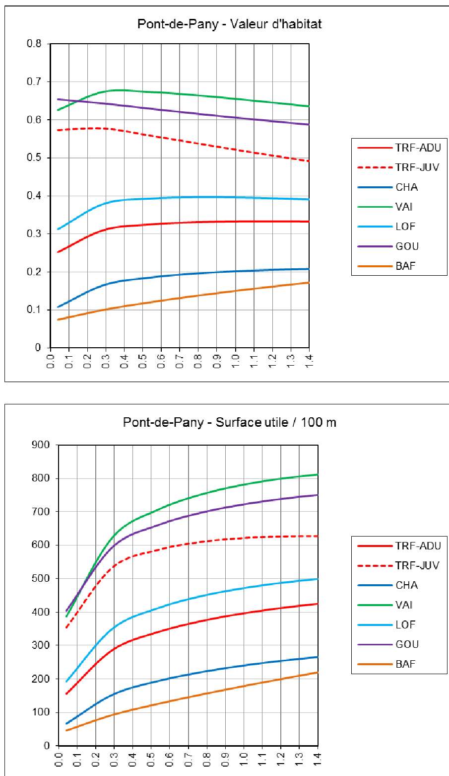
Figure 24 : Pont-de-Pany – Valeur d'habitat et surface utile par espèces (surface utile en m²/100 m en fonction du débit en m³/s)
