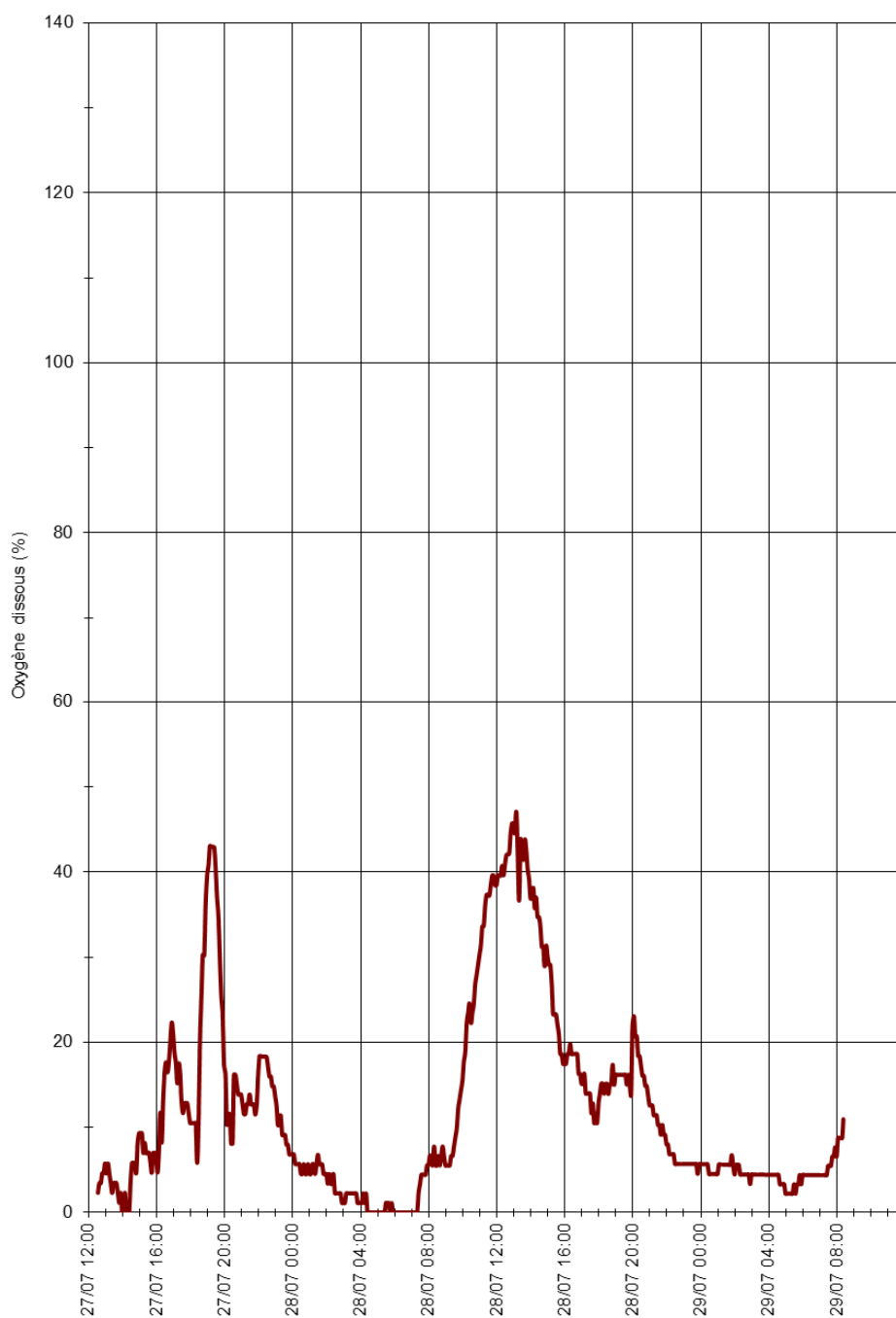
Figure 12 : Crimolois – Variations nycthémerales de la saturation en O2 – Juillet 2003
