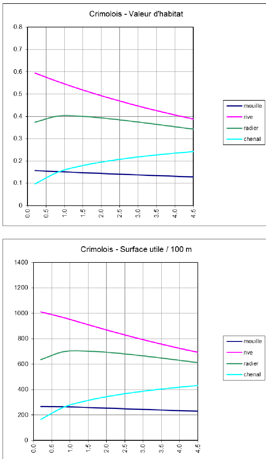
Figure 27 : Crimolois – Valeur d'habitat et surface utile par guild (surface utile en m^2/100\ m en fonction du débit en m^3/s )
