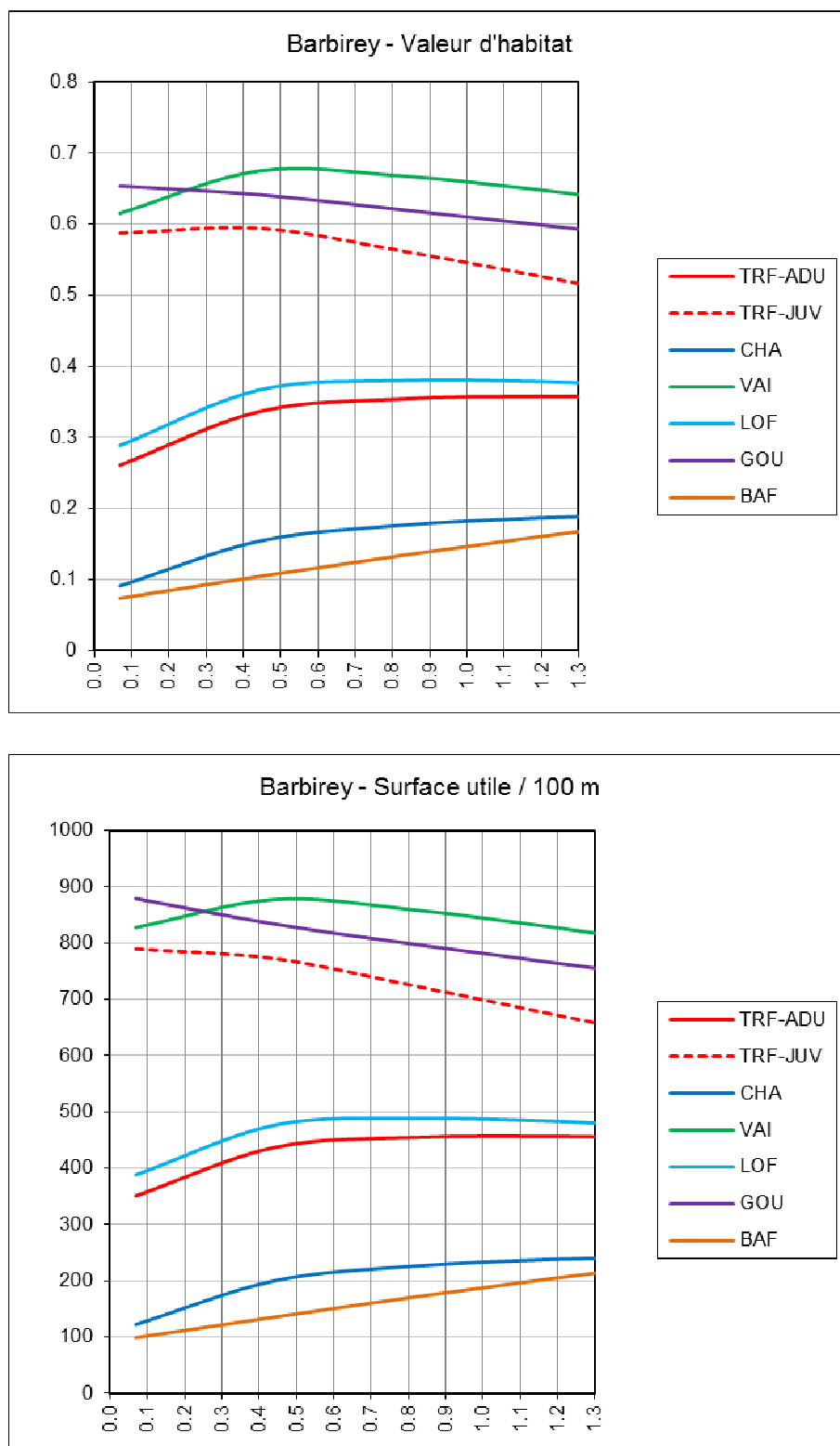
Figure 21 : Barbirey – Valeur d’habitat et surface utile par espèce (surface utile en m²/100 m en fonction du débit en m³/s)
