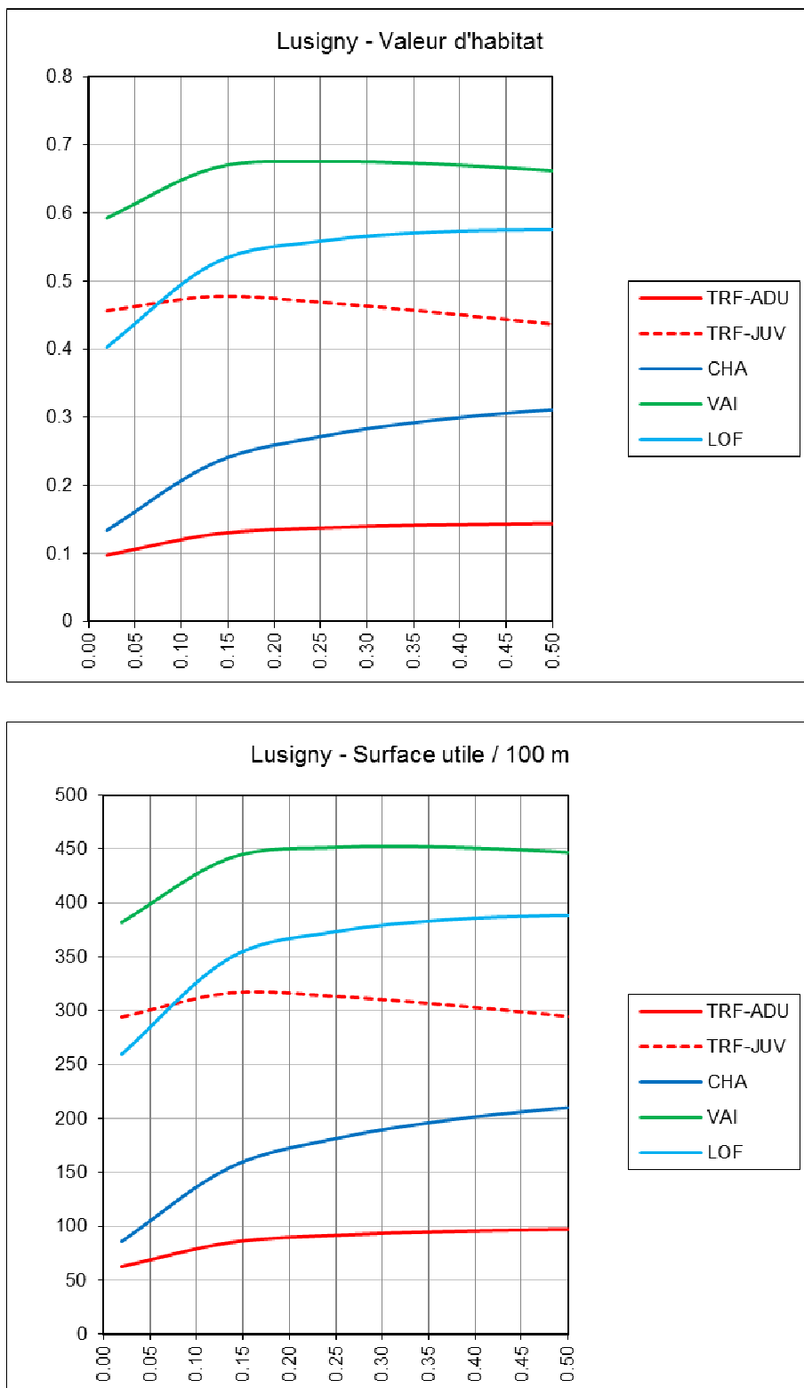
Figure 16 : Lusigny – Valeur d’habitat et surface utile par espèce (surface utile en m^2/100\text{ m} en fonction du débit en m^3/s )
