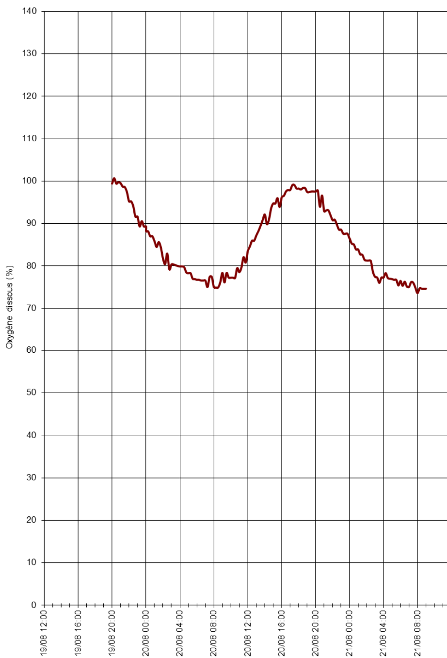
Figure 10 : Barbirey – Variations nycthémérales de la saturation en O2 – Août 2009
