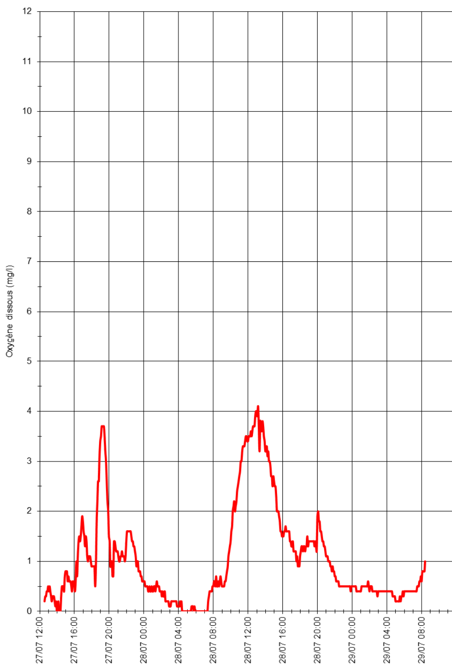
Figure 11 : Crimolois – Variations nycthémérales de l'oxygène dissous – Juillet 2003
