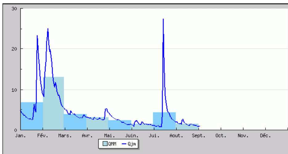
Figure 1 : Débits moyens journaliers à la station hydrométrique de Plombières – 2009 (Source DREAL Bourgogne – site hydroreel)
