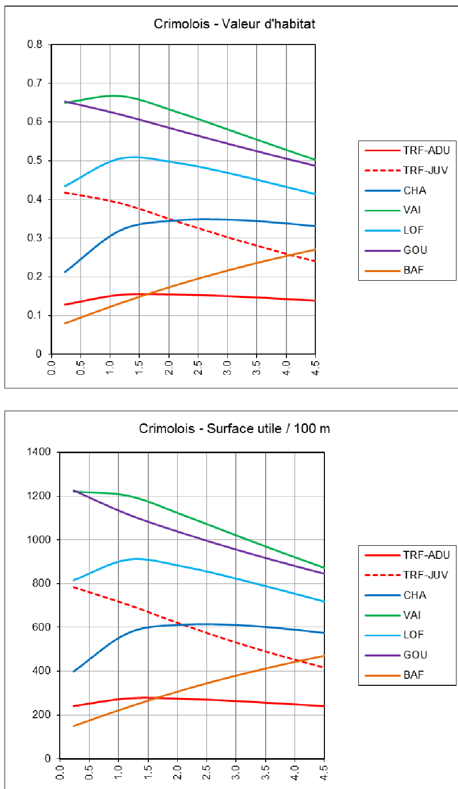
Figure 28 : Crimolois – Valeur d'habitat et surface utile par espèce (surface utile en m^2/100 m en fonction du débit en m^3/s )
