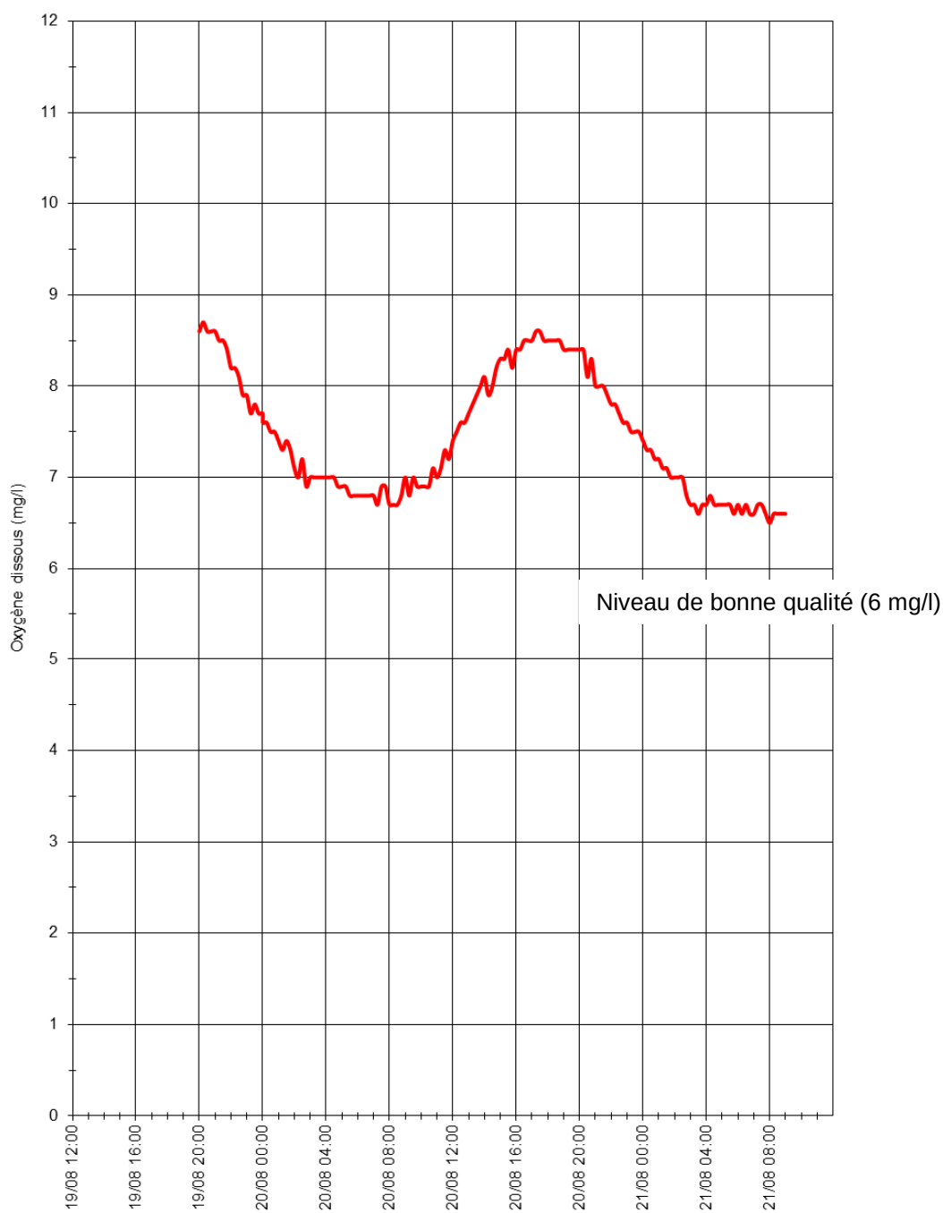
Figure 9 : Barbirey – Variations nycthémérales de l'oxygène dissous – Août 2009
