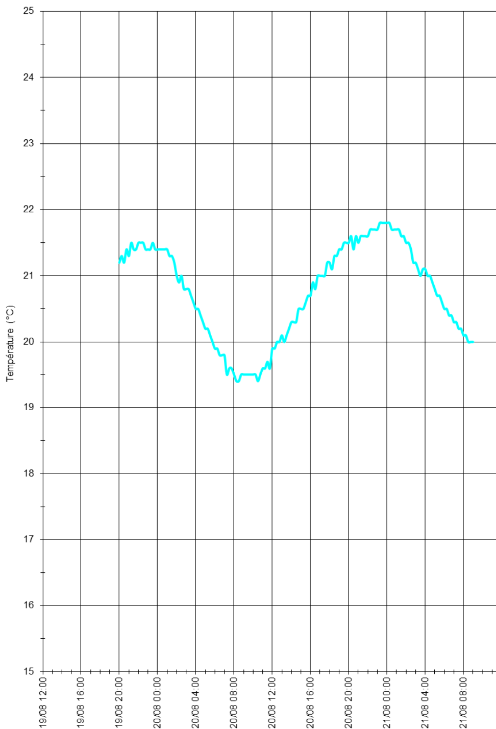
Figure 2 : Barbirey – Variations nycthémérales de la température – Août 2009
