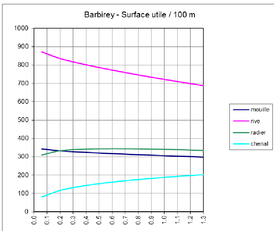
Figure 20 : Barbirey – Valeur d'habitat et surface utile par guild (surface utile en m^2/100 m en fonction du débit en m^3/s )
