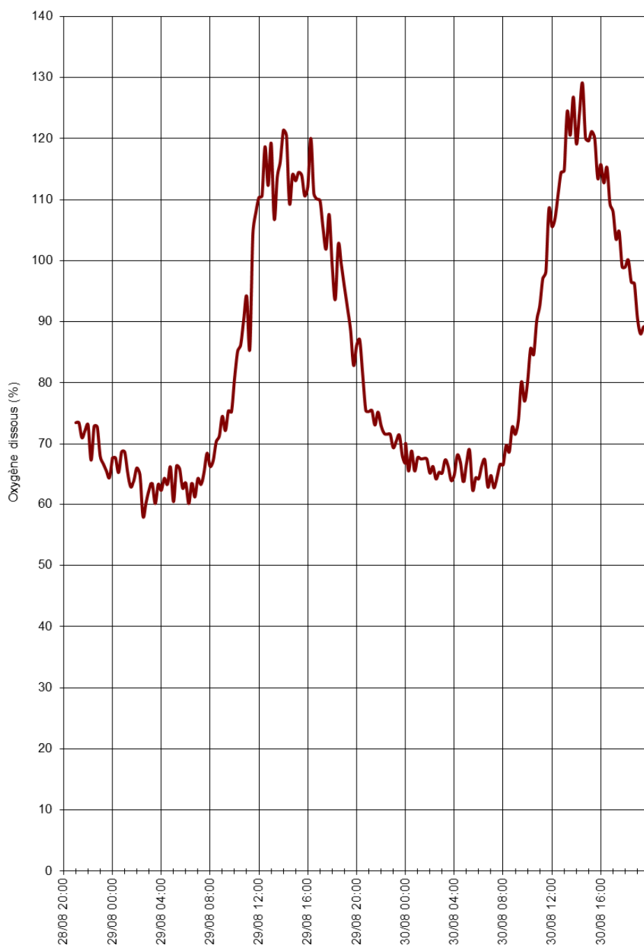
Figure 14 : Crimolois – Variations nycthémérales de la saturation en O2 – Août 2009
