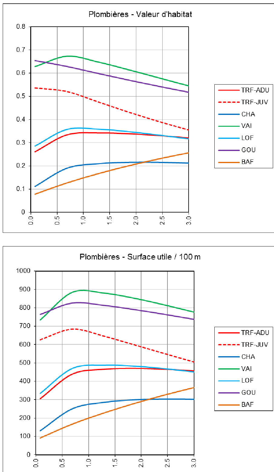
Figure 26 : Plombières – Valeur d'habitat et surface utile par espèces (surface utile en m^2/100\text{ m} en fonction du débit en m^3/s )
