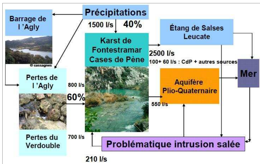
Figure 14: Schéma du bilan hydrologique du système karstique "Corbières d'Opoul et du synclinal Bas-Agly" - BRGM.
