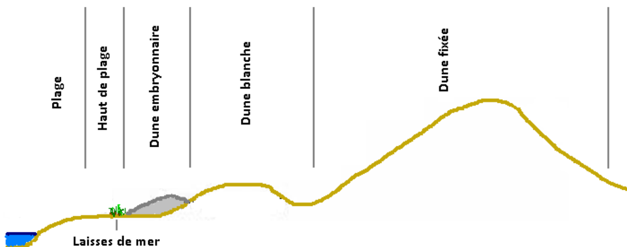
Figure 22 : Schéma type des lidos.
