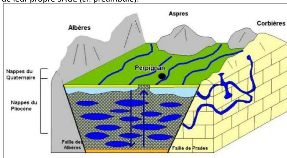
Figure 15 : Coupe schématique de la plaine du Roussillon sur sa partie aval 27 .
