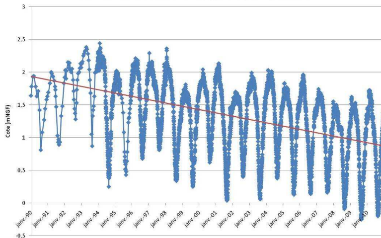
Figure 18 : Diminution chronique des nappes Pliocène au Barcarès
