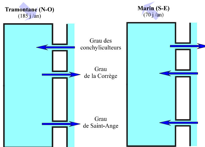
Figure 9 : fonctionnement schématique des graus en fonction des vents dominants.
