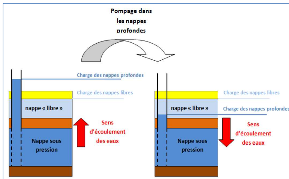
Figure 20 : Fonctionnement des phénomènes de drainance et d'inversion de drainance sur la partie aval 28
