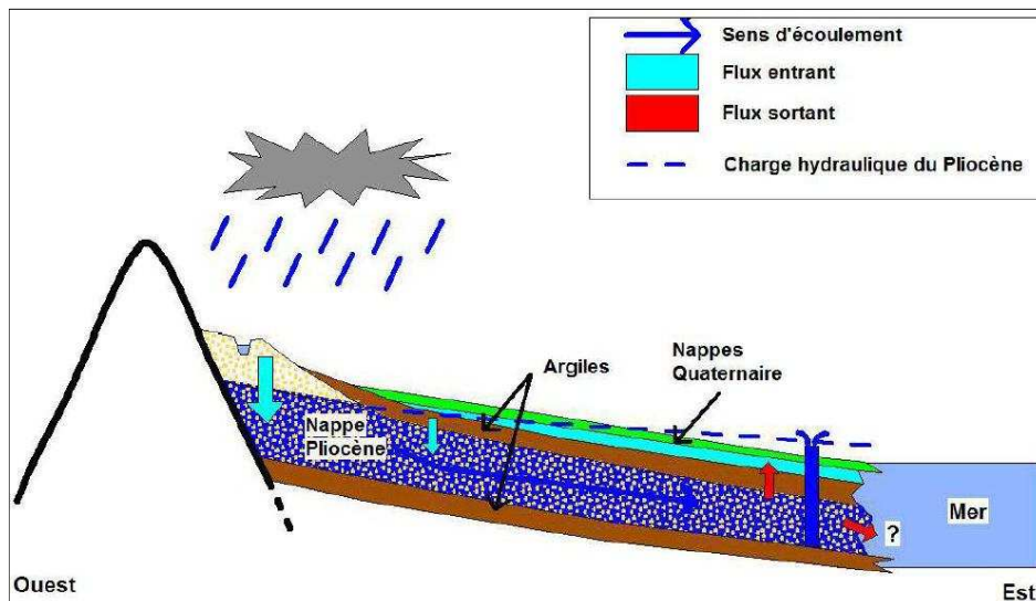
Figure 16: Coupe schématique du mode de fonctionnement des nappes Pliocène en l'état naturel 27 .
